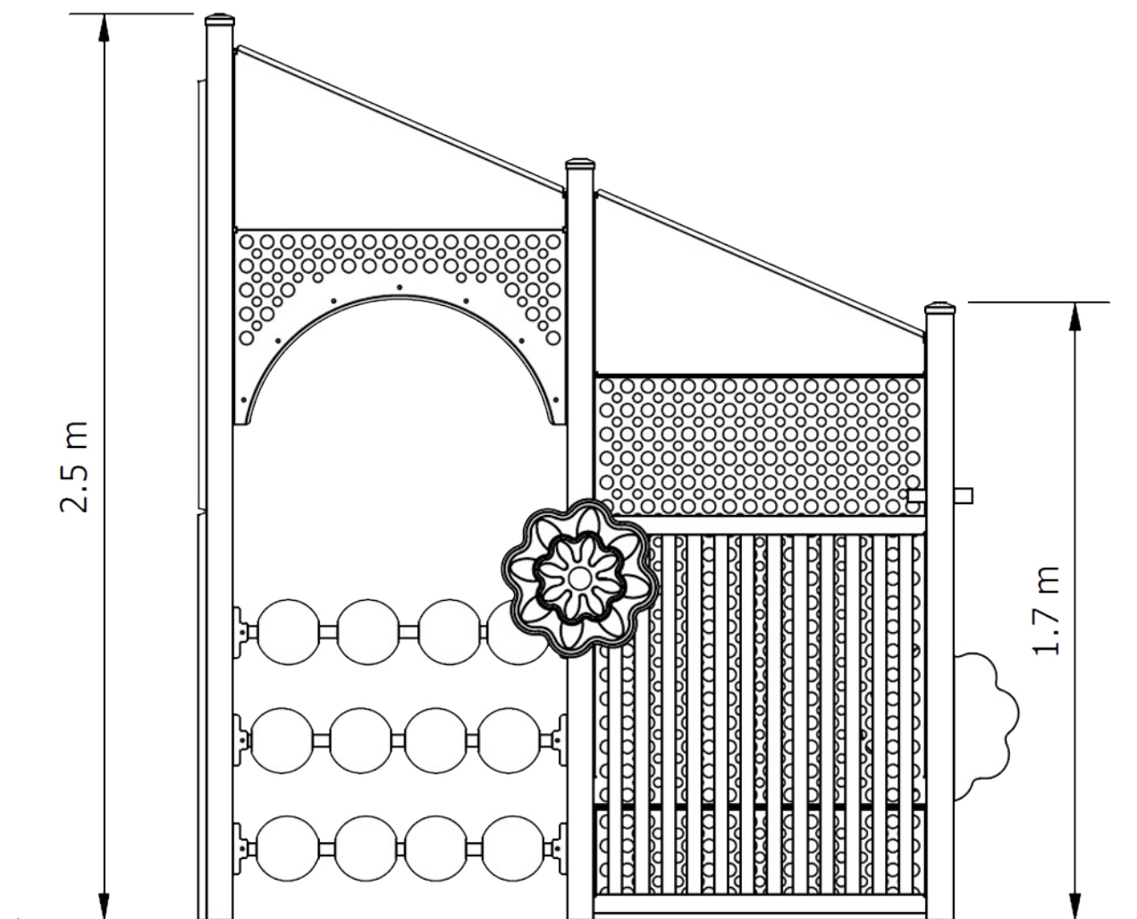
Elevation
